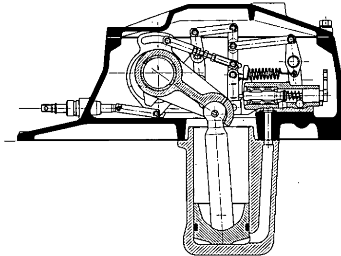
Fig. 212 - Asieme della Stazione Automatica di Controllo delle trattrici DELFINO 35 e AURORA 45 .
