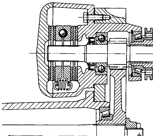
Fig. 178 - Sezione trasversale del gruppo freni delle trattrici SIRENETTA - DELFINO 35.
