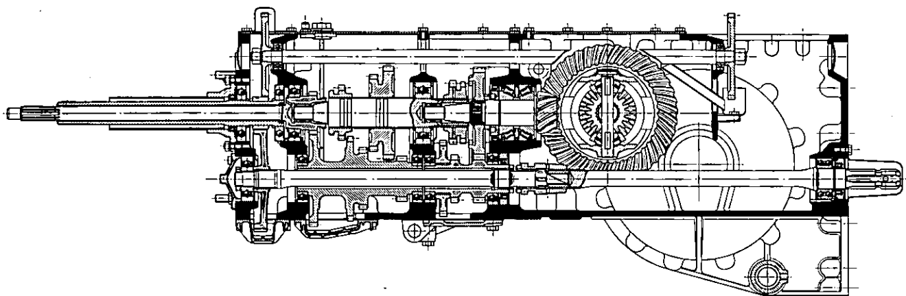
Fig. 102 - Sezione longitudinale del cambio delle trattrici Falcon , Minitauro 60 , Corsaro 70 e Saturno 80 .
