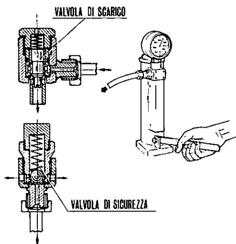
Fig. 208 - Controllo della taratura della valvola di sicurezza e della tenuta della valvola di scarico.
