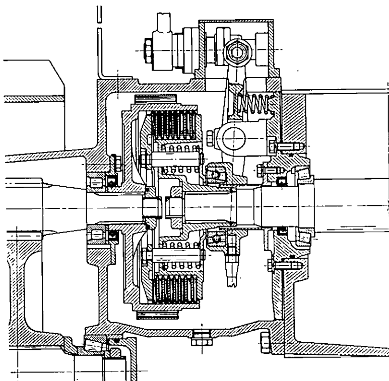
Fig. 91 - Gruppo comando frizione della trattrice Minitauro 60 C.
