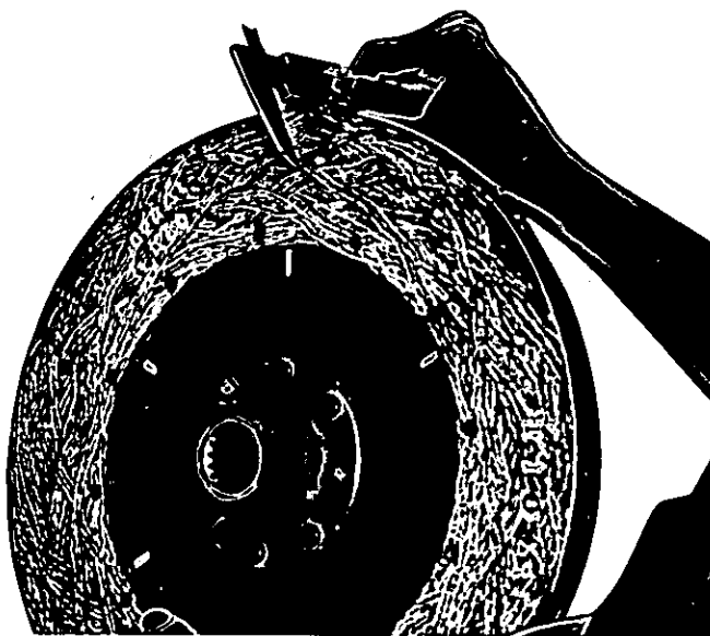
Fig. 64 - Misurazione dello spessore del disco frizione mediante il calibro 5.9030.271.0.
