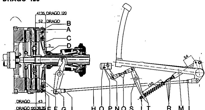
Fig. 73 - Gruppo comando frizione e freno-cambio delle trattrici Drago e Drago 120.
