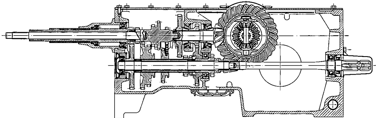
Fig. 98 - Sezione longitudinale del cambio della trattrice Delfino 35 .
