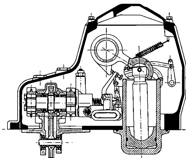
Fig. 224 - Assieme della Stazione Automatica di Controllo della trattoria DRAGO .
