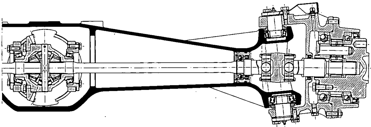
Fig. 139 - Assieme del complessivo trazione anteriore delle trattori Falcon e Minotauro 60 .
