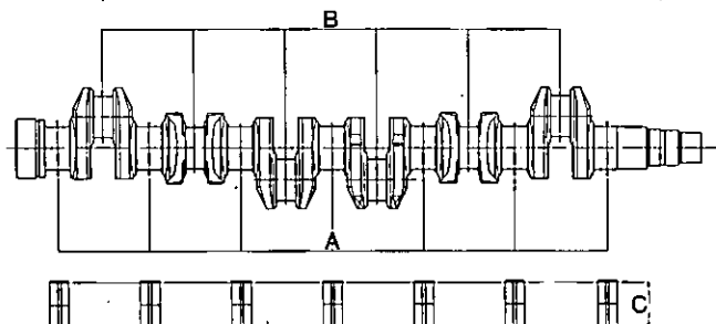
Fig. 13 - Dimensioni dei perni di banco e di biella dell'albero motore e dei semicuscinetti di banco e raggi dei perni dopo le rettifiche
