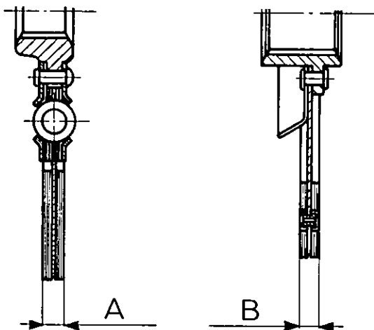
Fig. 63 - Spessore dei dischi frizione.
