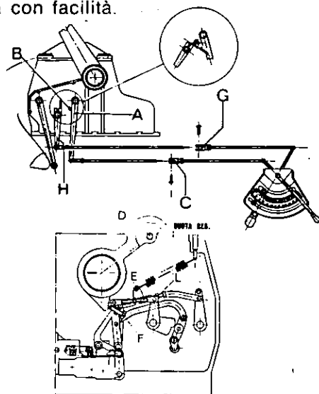
Fig. 226 - Schema di registrazione della Stazione Automatica di Controllo delle trattorie DRAGO e BUFFALO 120 .
