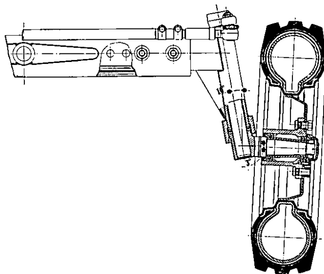
Fig. 133 - Assieme del gruppo assale anteriore della trattrice Buffalo 120.
