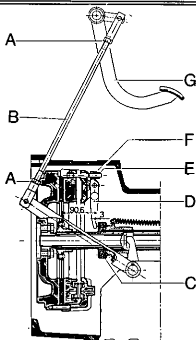
Fig. 72 - Gruppo comando frizione-cambio della trattrice Tiger 100.
