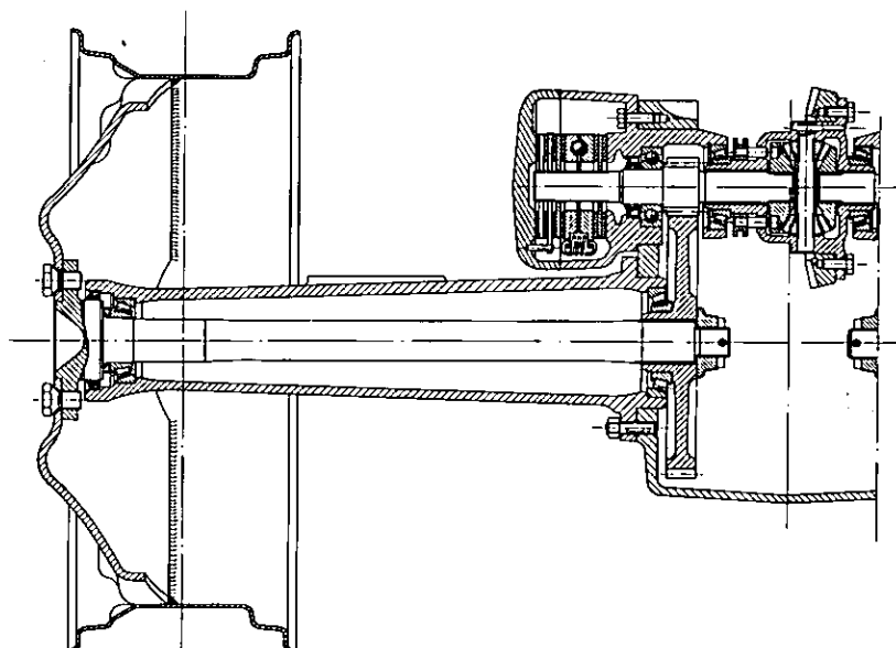
Fig. 108 - Sezione trasversale del cambio della trattrice Aurora 45 .
