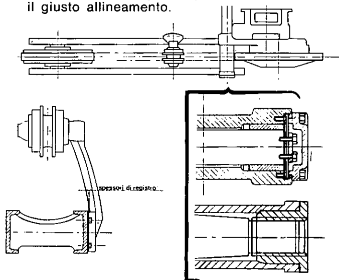
Fig. 190 - Allineamento tra ruota tendicingolo e rullo portacingolo e misurazione dell'allineamento del cingolo con la ruota motrice.
