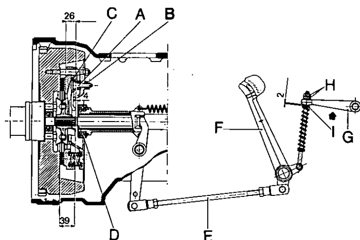
Fig. 65 - Gruppo comandi frizione e freno-cambio della trattrice Sirenetta.
