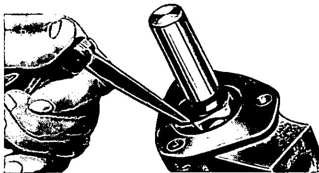
Fig. 94 - Controllo del gioco tra i rotori mediante lo spessore 5.9030.270.0.
