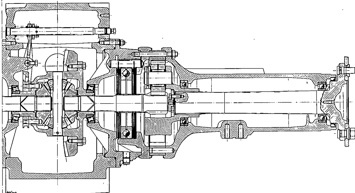
Fig. 113 - Sezione trasversale del cambio della trattrice Leopard 85 .
