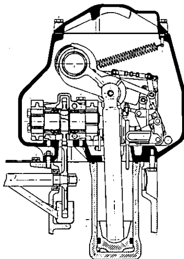
Fig. 218 - Asieme della Stazione Automatica di Controllo delle trattrici FALCON , MINITAURO 60 , CORSARO 70 e SATURNO 80 .
