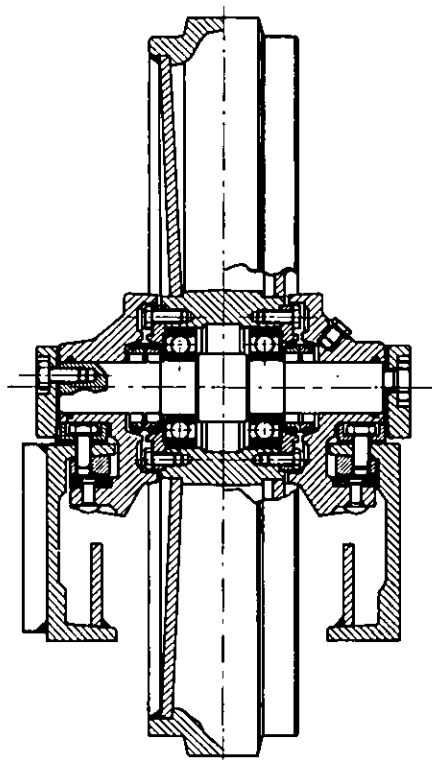
Fig. 193 - Schema d'assieme della ruota tendicingolo per FALCON C.
