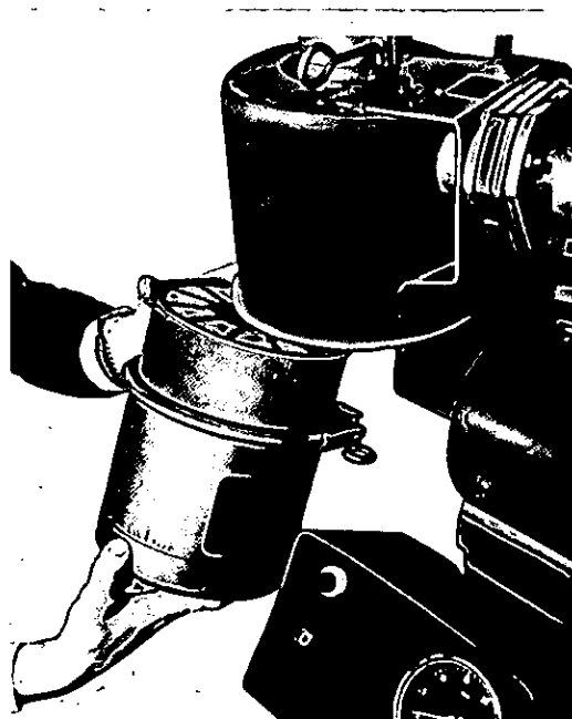
Fig. 62 - Pulizia filtro bagno olio
