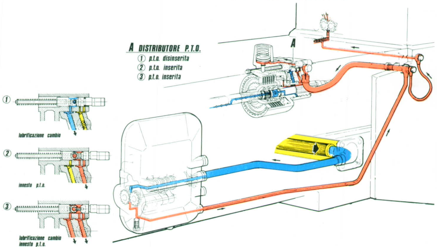
Fig. 78 - Gruppo frizione della P.T.O.
