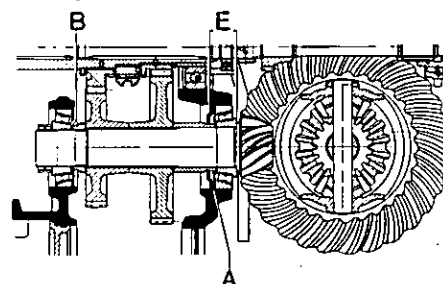
Fig. 121 - Coppia conica della trattrice Drago e Drago 120.
