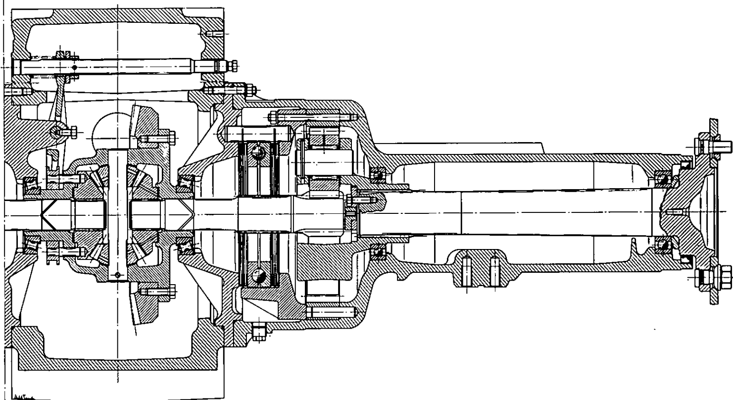
Fig. 114 - Sezione trasversale del cambio delle trattrici Panther e Panther 90 .
