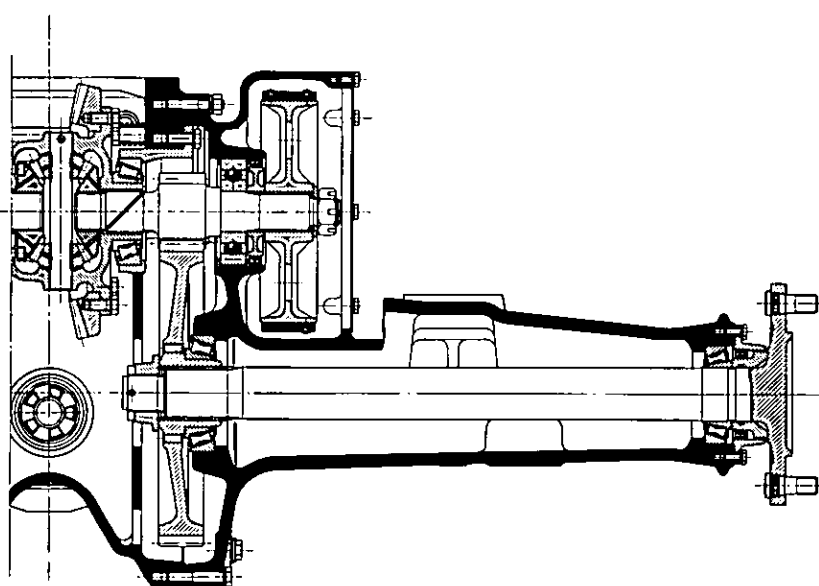
Fig. 110 - Sezione trasversale del cambio della trattrice Minitauro 60 C .
