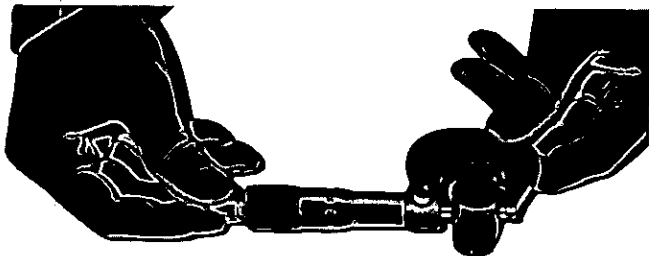
Fig. 201 - Controllo del diametro degli stantuffi della pompa idraulica radiale mediante il calibro micrometrico 5.9030.368.0.
