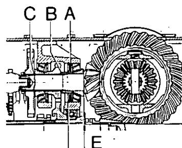
Fig. 117. Coppia conica delle trattrici Sirenetta e Delfino 35
