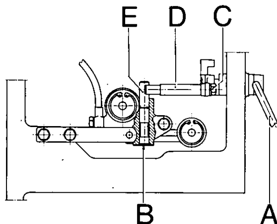
Fig. 80 - Gruppo comando distributore idraulico.
