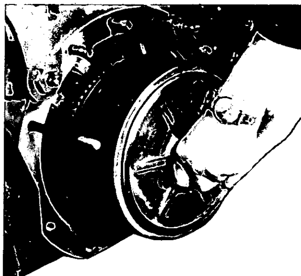
Fig. 89 - Allineamento dei dischi frizione con il tamburo dei freni a nastro.
