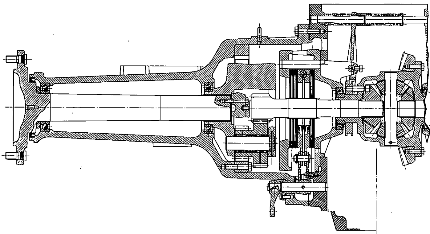
Fig. 116 - Sezione trasversale del cambio delle trattrici Dragor, Dragor 120, Buffalo 120 e Buffalo 130 .
