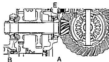
Fig. 122 - Coppia conica delle trattrici Buffalo 120 e Buffalo 130.
