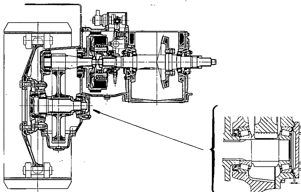
Fig. 110 - Sezione trasversale del cambio della trattrice Minitauro 60 C .
