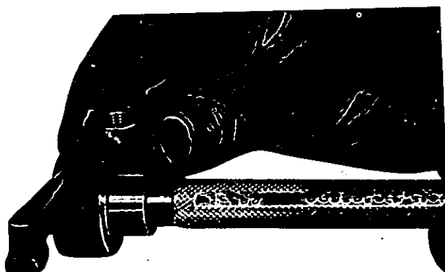
Fig. 8 - Controllo del diametro interno delle boccole dei bilancieri mediante calibro a tamponi 5.9030.369.0
