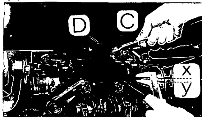
Fig. 216 - Registrazione della corsa massima dei bracci di sollevamento.
