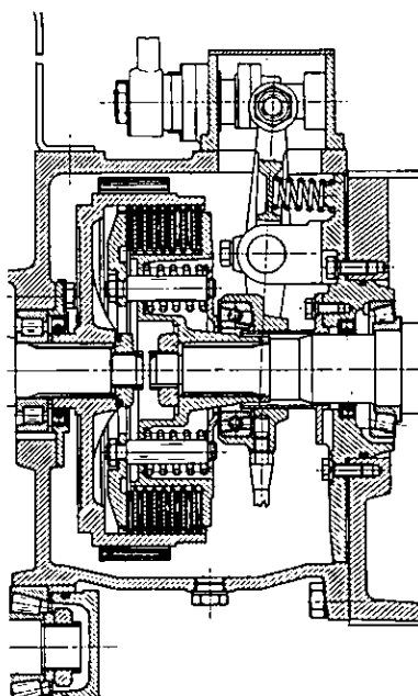
Fig. 182 - Sezione trasversale del gruppo freni della trattore MINITAURO 60 C.
