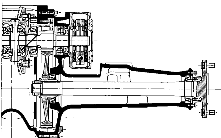
Fig. 112 - Sezione trasversale del cambio della trattrice Saturno 80 .
