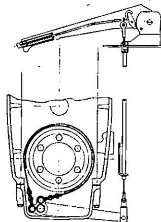
Fig. 176 - Assieme dei comandi del freno a nastro di stazionamento per Trattorice TIGER 100 .
