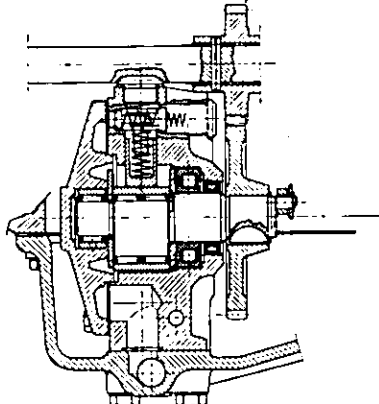
Fig. 196 - Pompa a pistoni radiali SAME per trattrici LEOPARD 85 - PANTHER - PANTHER 90 e TIGER 100.
