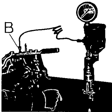
Fig. 204 - Controllo della tenuta della pompa SAC delle trattrici PANTHER e TIGER 100 mediante attrezzo 5.9030.463.0.
