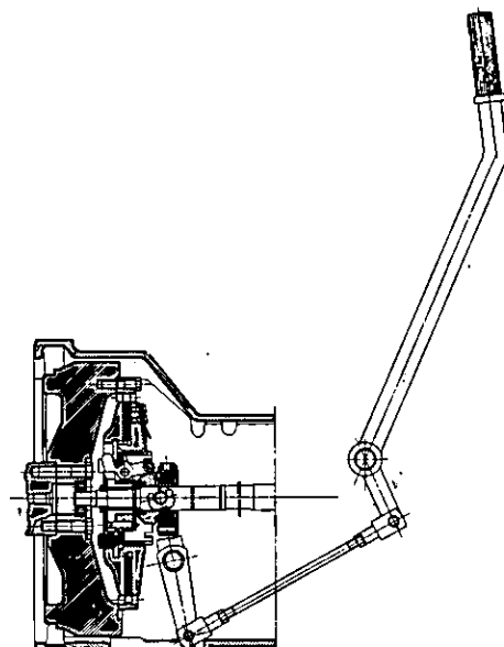
Fig. 84 - Gruppo comando frizione della trattrice Falcon C.
