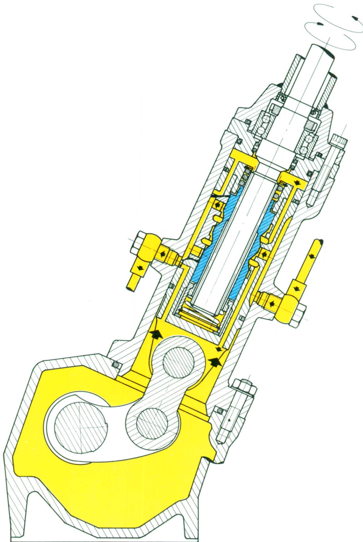
Fig. 156 - Posizione di fine corsa superiore.
