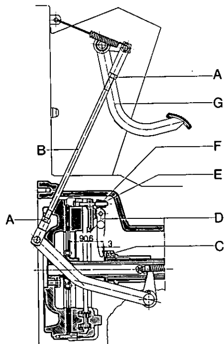
Fig. 75 - Gruppo comando frizione-cambio della trattoria Buffalo 130.
