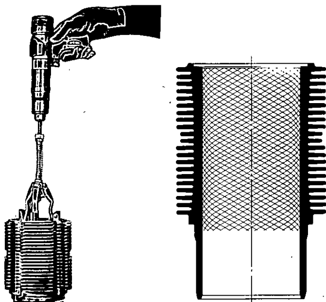
Fig. 33 - Ripassatura dei cilindri mediante l'attrezzo 5.9030.349.0
