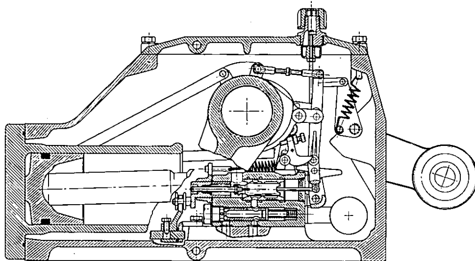
Fig. 222 - Assieme della Stazione Automatica di Controllo delle trattrici LEOPARD 85, PANTHER 90 e TIGER 100.
