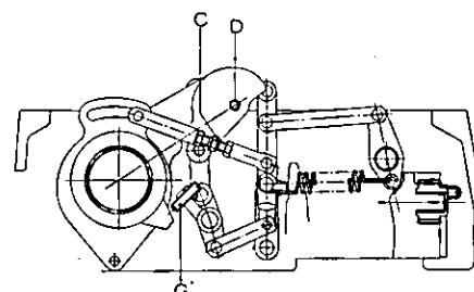
Fig. 213 - Schema di registrazione della Stazione Automatica di Controllo delle trattrici DELFINO 35 e AURORA 45 .
