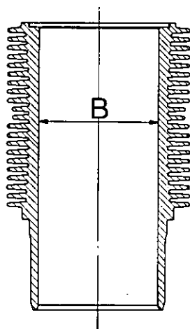
Fig. 32 - Diametro del cilindro
