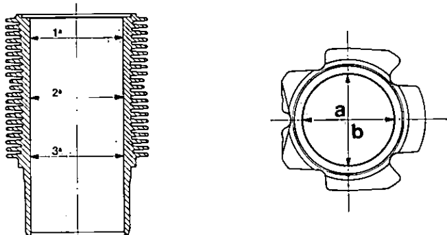
Fig. 31. - Schema per il controllo dei cilindri
