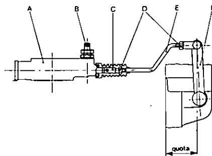
Fig. 42 b - Collegamento della pompa d'iniezione al regolatore
