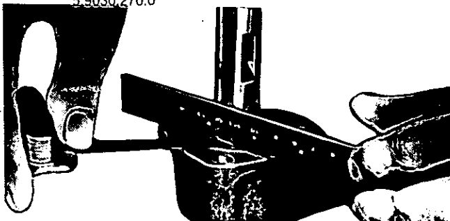
Fig. 96 - Controllo del gioco tra il lato superiore ed il piano di appoggio del corpo della pompa.
