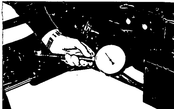
Fig. 162 - Controllo della taratura della valvola di sicurezza con manometro 5.9030.274.0 e raccordo 5.9030.447.0.
