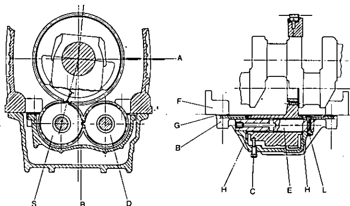
Fig. 34 b - Registrazione e messa in fase delle masse controrotanti
