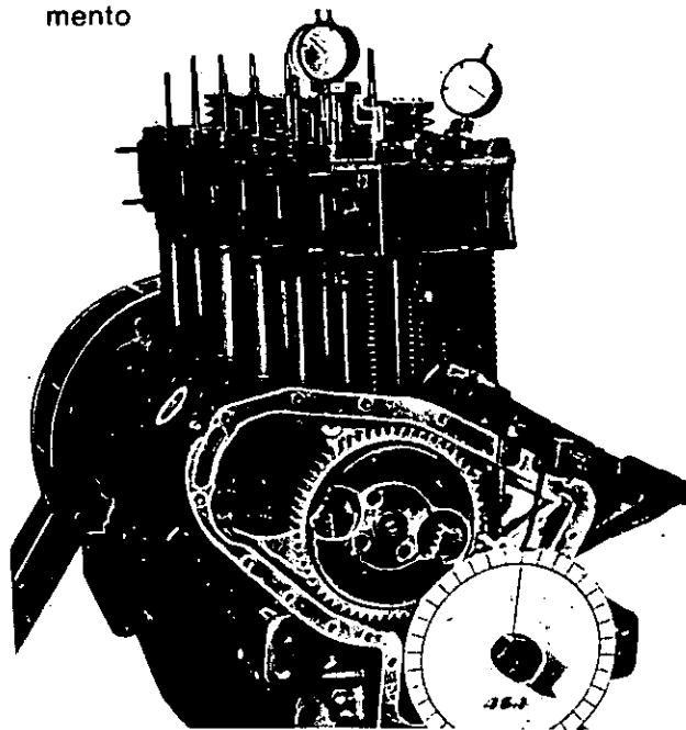
Fig. 18 - Bilanciamento della distribuzione
