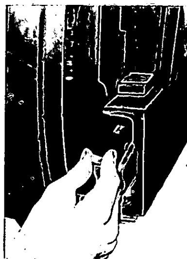
Fig. 191 - Registrazione del gioco assiale della ruota tendicingolo con spessimetro 5.9030.270.0
