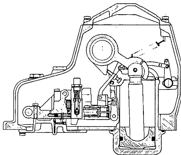
Fig. 225 - Assieme della Stazione Automatica di Controllo della trattoria BUFFALO 120 .
