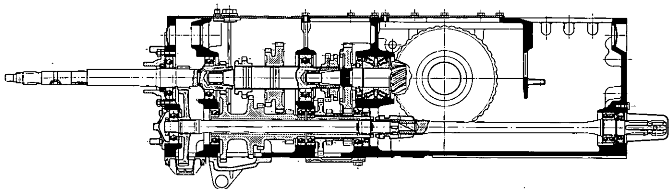
Fig. 101 Sezione longitudinale del cambio della trattrice Minitauro 60 C .
