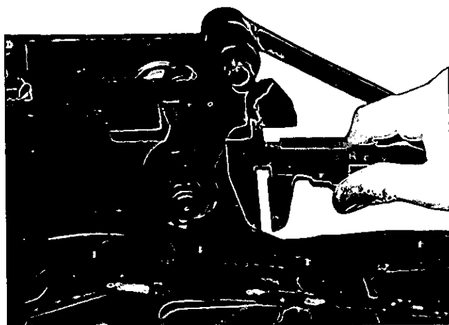
Fig. 92 - Misurazione della corsa a vuoto della leva di comando frizione.
