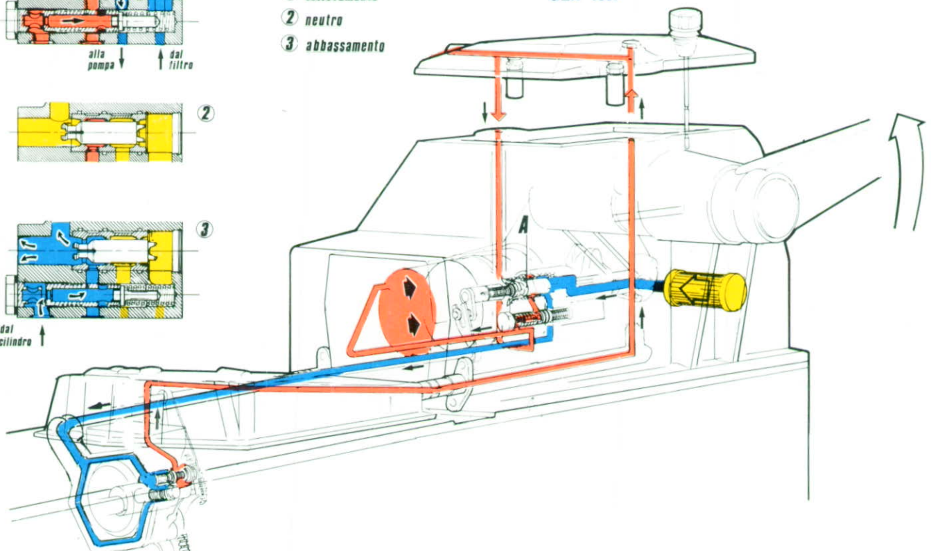
Fig. 235 - Schema di funzionamento del circuito idraulico della Stazione Automatica di Controllo delle trattori LEOPARD 85, PANTHER, PANTHER 90 e TIGER 100.
