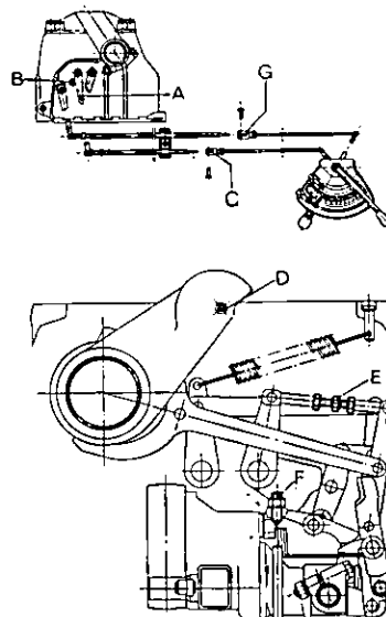
Fig. 219 - Schema di registrazione della Stazione Automatica di Controllo delle trattrici FALCON , MINITAURO 60 , CORSARO 70 e SATURNO 80 .
