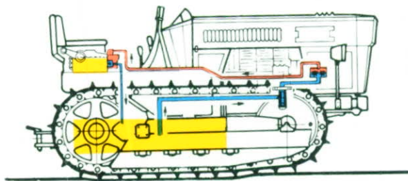
Fig. 232 - Schema di funzionamento della Stazione Automatica di Controllo della trattore FALCON C (dalla matr. 4145).
