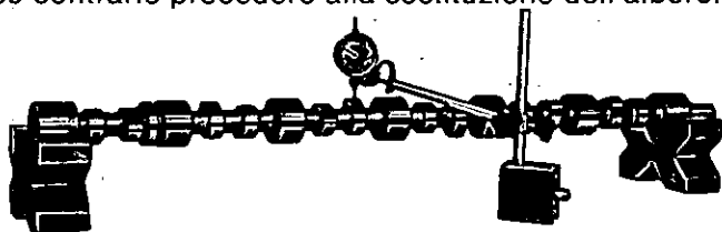
Fig. 17 - Controllo dell'alzata degli eccentrici dell'albero della distribuzione, mediante il comparatore centesimale 5.9030.272.0 e la base magnetica 5.9030.267.0
