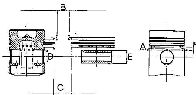
Fig. 24 - Diametri e giochi dei pistoni e delle fasce elastiche
