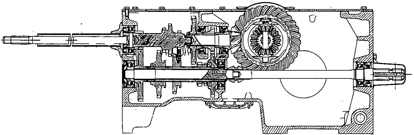
Fig. 97 - Sezione longitudinale del cambio della trattrice Sirenna .
