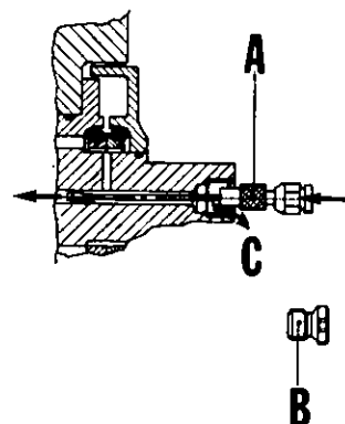
Fig. 188 - Lubrificazione dei rulli di guida e della ruota tendicingolo.
