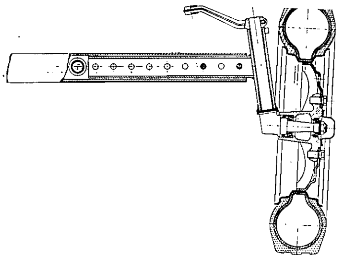
Fig. 129 - Assieme del gruppo assale anteriore delle trattrici Sirenella , Delfino 35 e Aurora 45 .
