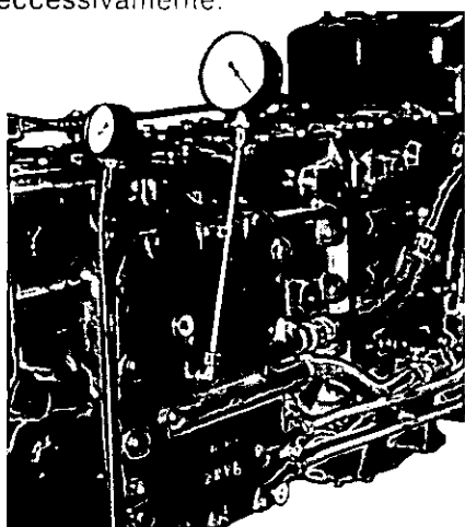
Fig. 203 - Controllo della tenuta del circuito idraulico mediante vuotometro per trattori BUFFALO 120 e BUFFALO 130 .
