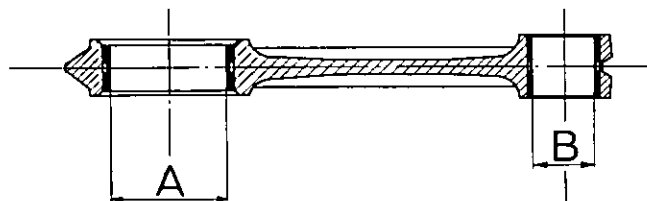
Fig. 21 - Dimensioni delle bielle e relative boccole
