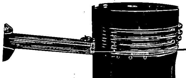
Fig. 26 - Misurazione del gioco tra fasce elastiche e relative sedi, mediante lo spessore 5.9030.270.0
