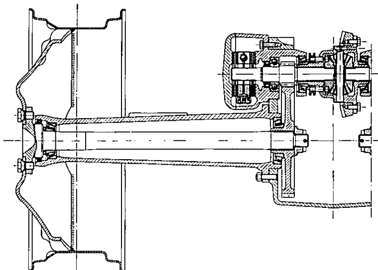
Fig 107 - Sezione trasversale del cambio delle trattrici Sirenetta , Delfino 35 .
