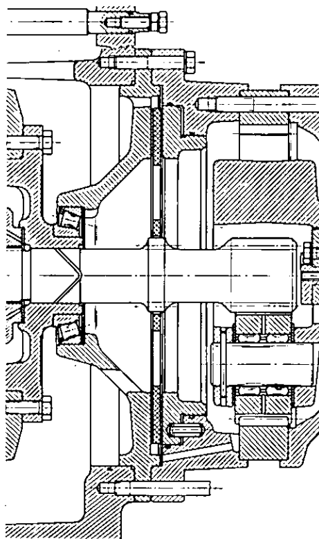
Fig. 184 - Sezione trasversale del gruppo freni della trattrice TIGER 100.
