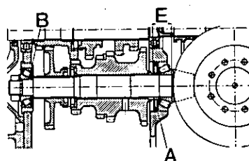
Fig. 118 - Coppia conica della trattrice Falcon C.
