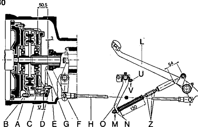
Fig. 70 - Gruppo comando frizioni e freno-cambio delle trattrici Corsaro 70 e Saturno 80.
