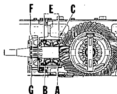
Fig. 124 - Coppia conica delle trattrici Corsaro 70, Saturno 80.
