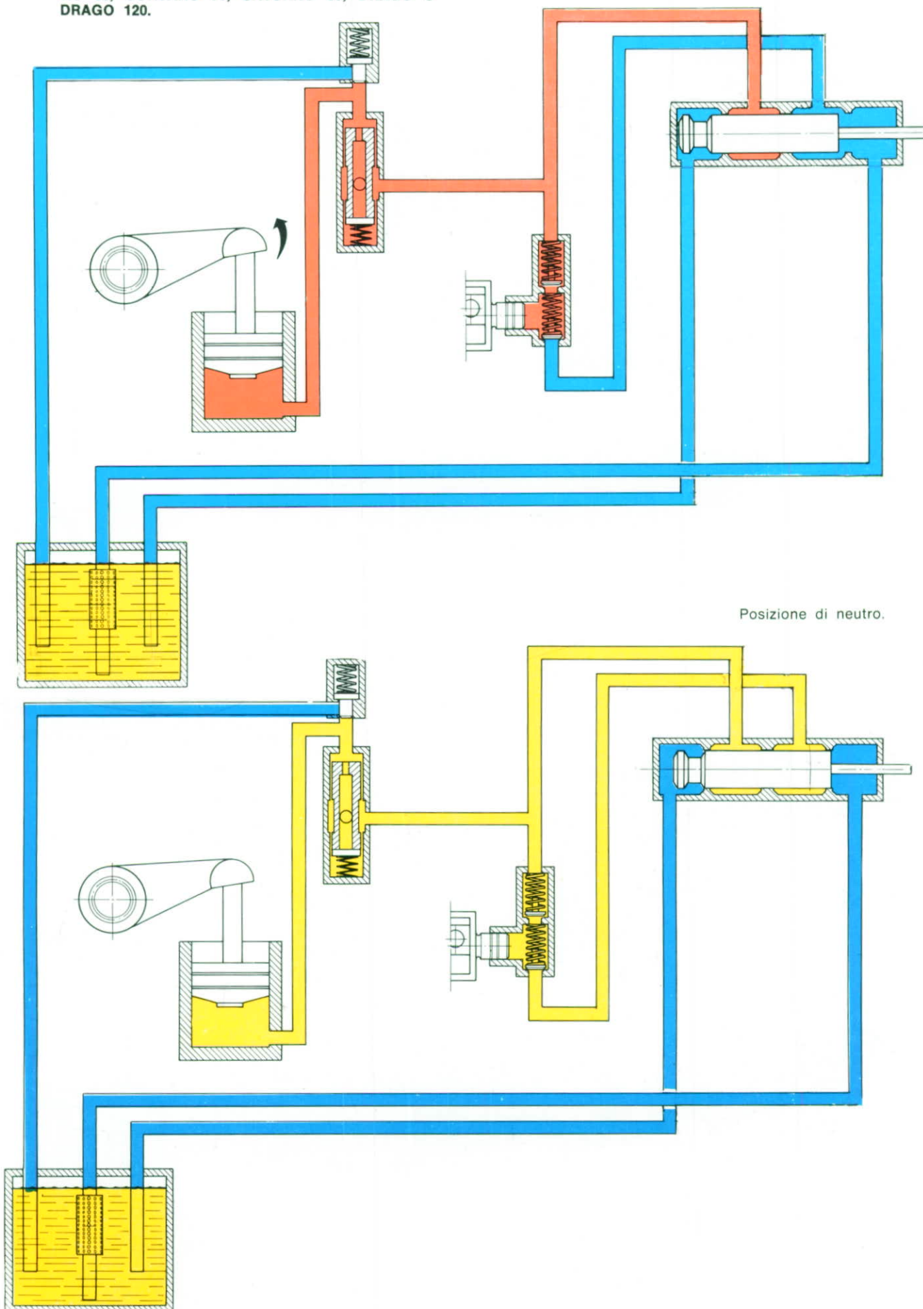
Fig. 234 - Schema di funzionamento della Stazione Automatica di Controllo delle Trattori FALCON , MINITAURO 60, CORSARO 70, SATURNO 80, DRAGO e DRAGO 120.
