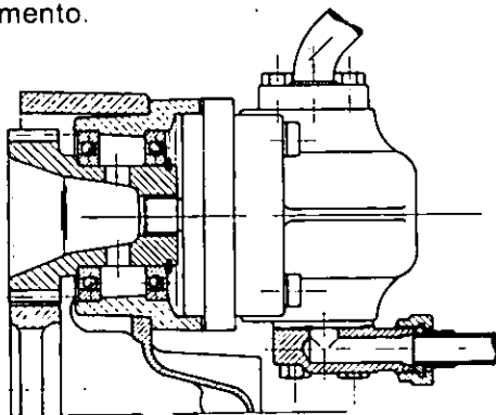
Fig. 195 - Pompa ad ingranaggi BOSCH per trattrici SIRENETTA, DELFINO 35, AURORA 45, FALCON C e MINITAURO 60 C.
