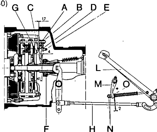
Fig. 68 - Gruppo comandi frizioni e freno-cambio della trattrice Falcon (fino alla matricola n. 3240).
