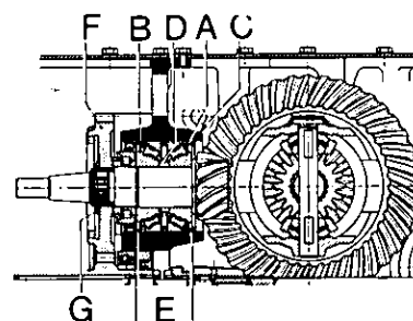
Fig. 123 - Coppia conica delle trattrici Falcon, Minitauro 60, Minitauro 60 C.
