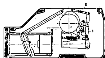
Fig. 223 - Schema di registrazione della Stazione Automatica di Controllo delle trattrici LEOPARD 85, PANTHER 90, TIGER 100.
