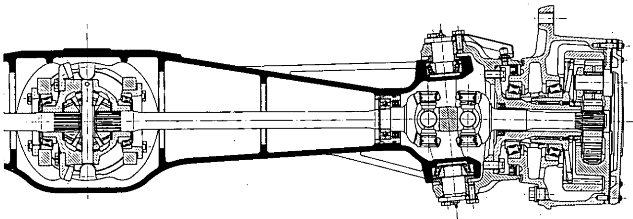
Fig. 140 - Assieme del complessivo trazione anteriore delle trattori Corsaro 70 , Saturno 80 e Leopard 85 .
