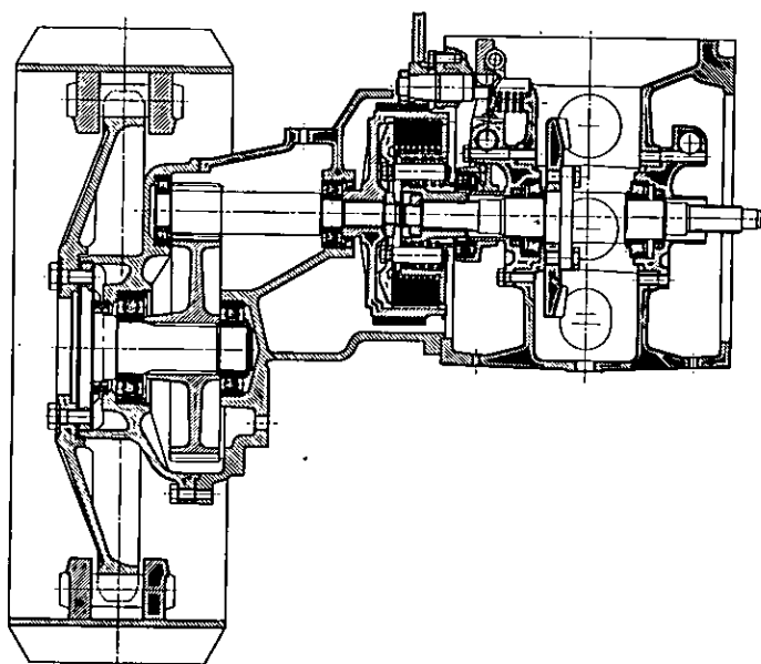
Fig. 109 - Sezione trasversale del cambio della trattrice Falcon C .
