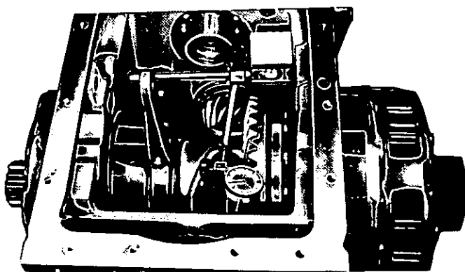
Fig. 125 - Misurazione del gioco tra i denti del pignone e della corona conica, mediante il comparatore 5.9030.270.0 e la base magnetica 5.9030.267.0.
