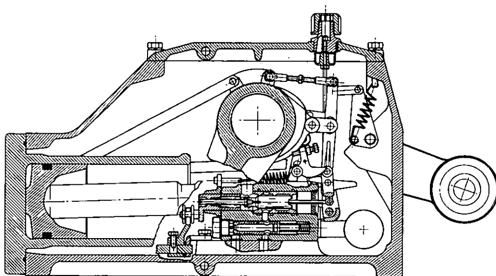
Fig. 220 - Assieme della Stazione Automatica di Controllo della trattrice PANTHER .
