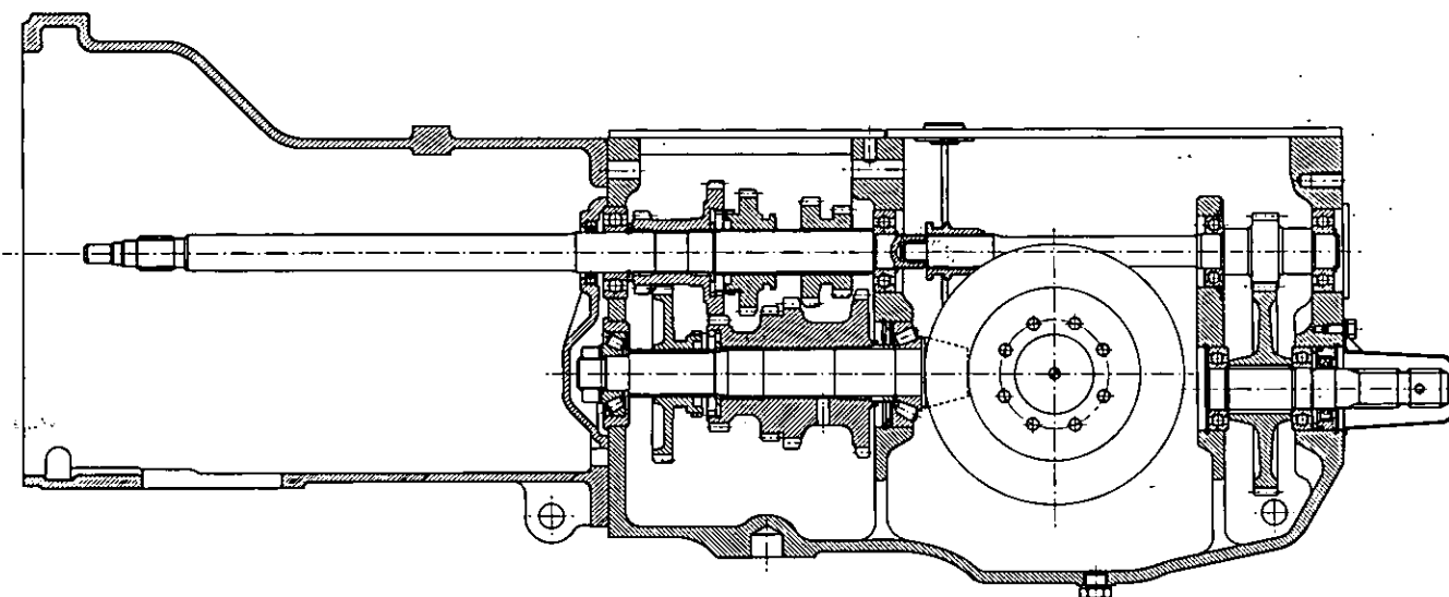
Fig. 100 Sezione longitudinale del cambio della trattrice Falcon C .
