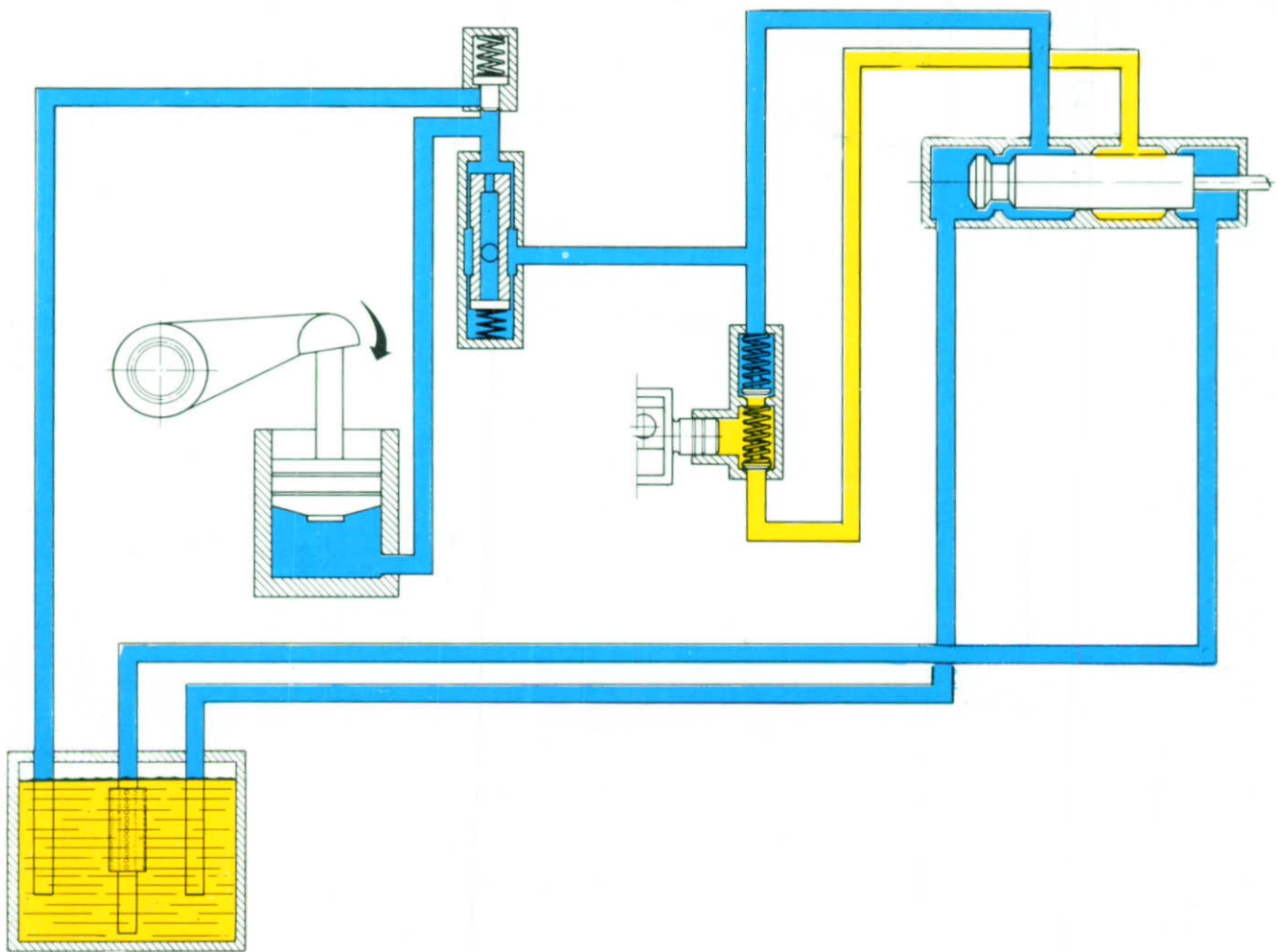
Fig. 235 - Schema di funzionamento del circuito idraulico della Stazione Automatica di Controllo delle trattori LEOPARD 85, PANTHER, PANTHER 90 e TIGER 100.
