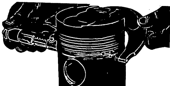
Fig. 23 - Misurazione del diametro del pistone, mediante il calibro micrometrico
