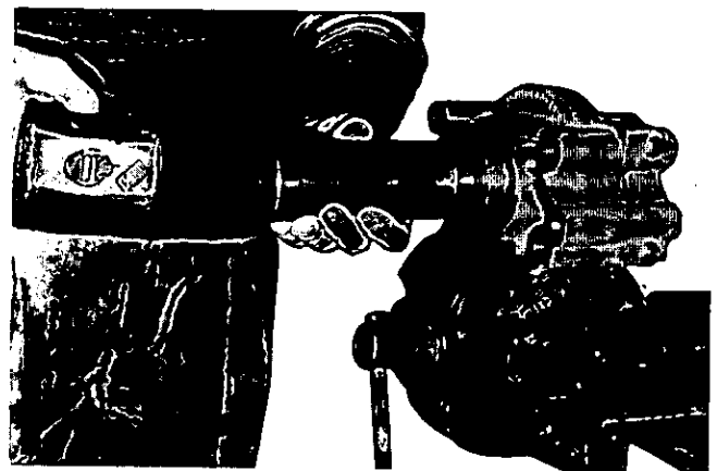
Fig. 207 - Montaggio degli anelli di tenuta mediante l'attrezzatura 5.9030.421.0.
