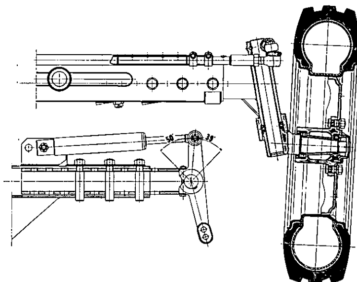
Fig. 132 - Assieme del gruppo assale anteriore delle trattrici Panther 90. Tiger 100. Buffalo 130.
