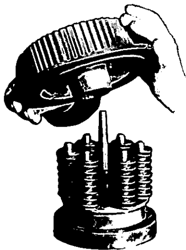
Fig. 86 - Smontaggio del gruppo frizione mediante l'attrezzo 5.9030.468.0.
