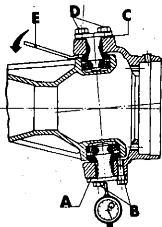
Fig. 137 - Misurazione del gioco dei forcelloni mediante il comparatore 5.9030.272.0 e base magnetica 5.9030.267.0.
