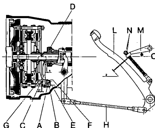
Fig. 67 - Gruppo comandi frizioni e freno-cambio della trattrice Aurora 45.
