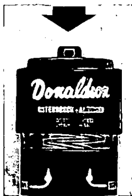
Fig. 55 - Spia meccanica di intasamento - Pulsante per il ritorno del segnale rosso
