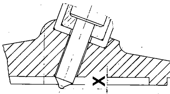
Fig. 51 b - Sporgenza degli iniettori dal piano della testa
