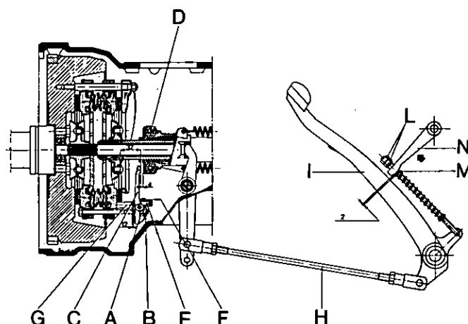
Fig. 66 - Gruppo comandi frizioni e freno-cambio della trattrice Delfino 35.
