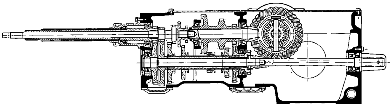
Fig. 99 - Sezione longitudinale del cambio della trattrice Aurora 45 .
