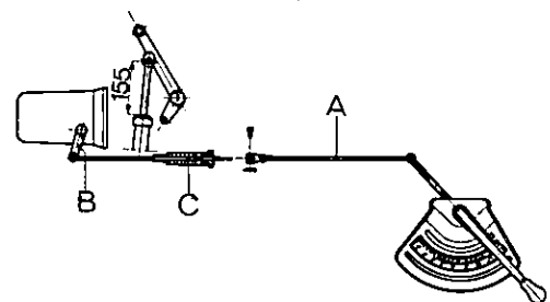
Fig. 210 - Assieme della Stazione Automatica di Controllo delle trattrici SIRENETTA e FALCON C (fino alla matr. 4144).
