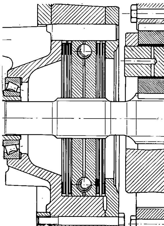
Fig. 185 - Sezione trasversale del gruppo freni delle trattrici LEOPARD 85, PANTHER, PANTHER 90, DRAGO e DRAGO 120.
