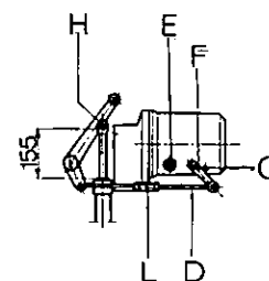
Fig. 211 - Schema di registrazione dalla Stazione Automatica di Controllo delle trattrici SIRENETTA e FALCON C (fino alla matr. 4144).
