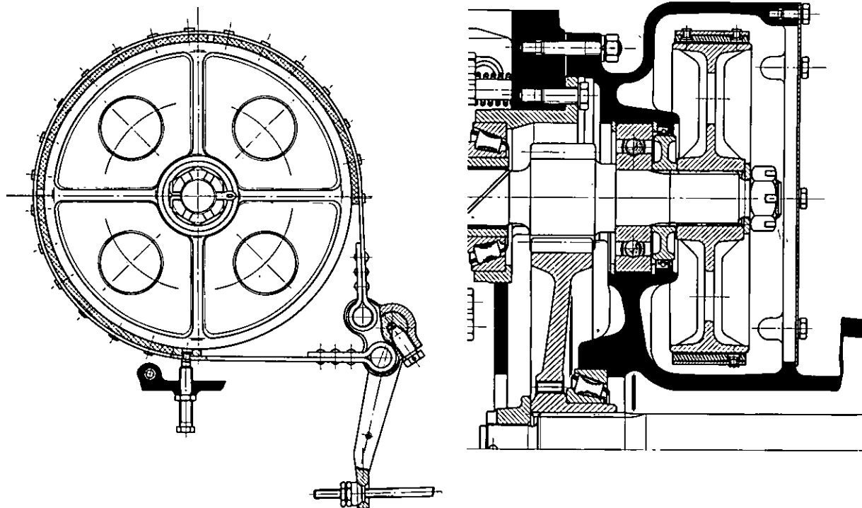
Fig. 180 - Sezione trasversale del gruppo freni delle trattori FALCON - MINITAURO 60 e CORSARO 70.
